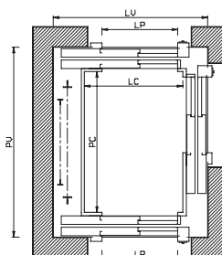
3 accessi
