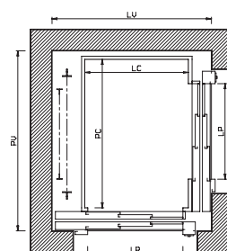
2 accessi adiacenti
