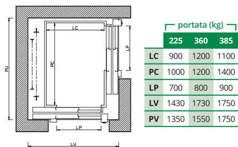
2 accessi adiacenti
