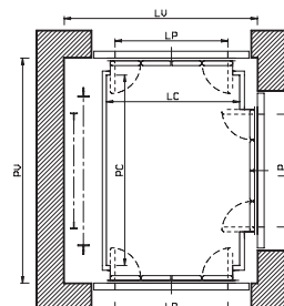
3 accessi
