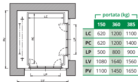
2 accessi adiacenti
